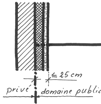
Figure 3 : Isolation thermique sur le domaine public
