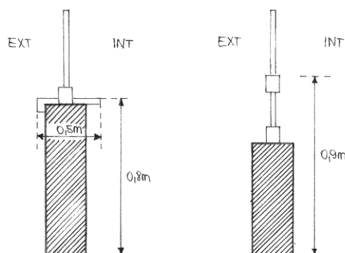
Figure 16 : hauteurs allèges
