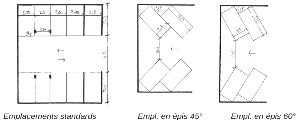
Figure 6 : dimensionnement des emplacements pour voitures
