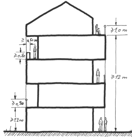
Figure 14 : hauteur des garde-corps
